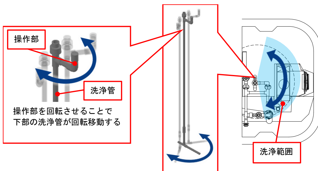
可動式洗浄管の構造と洗浄範囲(5, 7 人槽)
