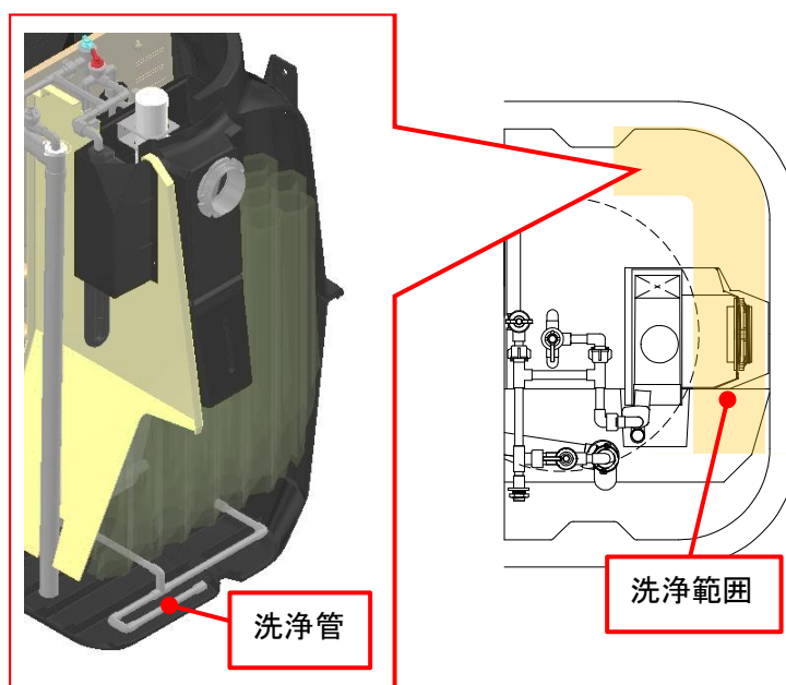
固定式洗浄管の構造と洗浄範囲(5, 7 人槽)
