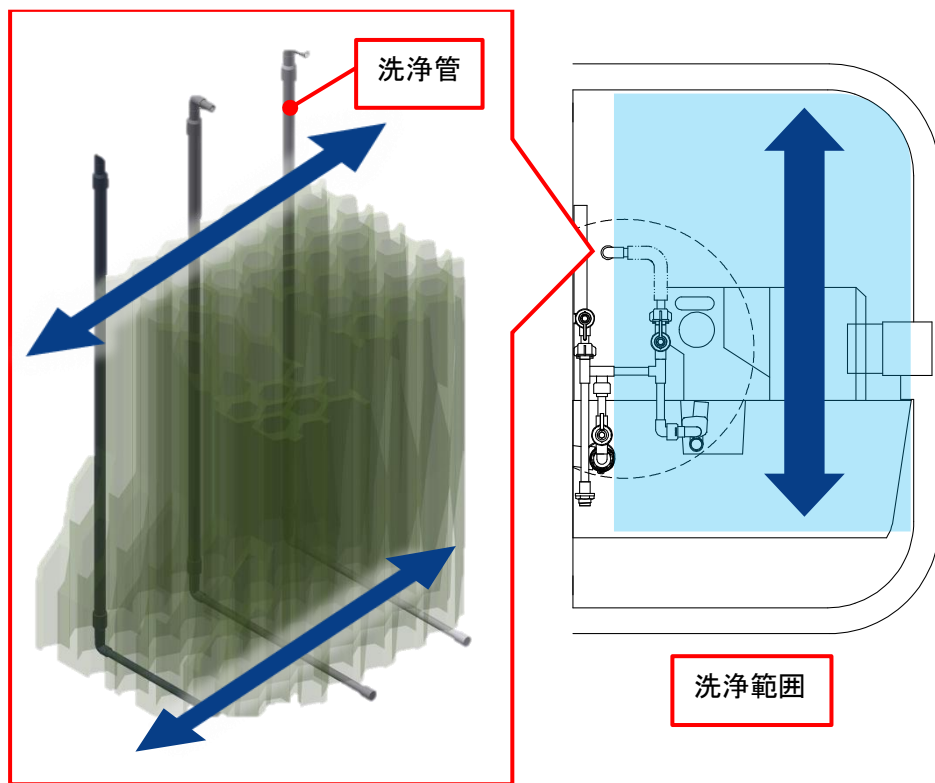
可動式洗淨管の構造と洗淨範囲(10 人槽)
