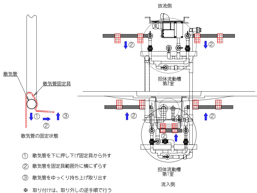
図 3 - 2 散気装置の固定状態および取り外し方
