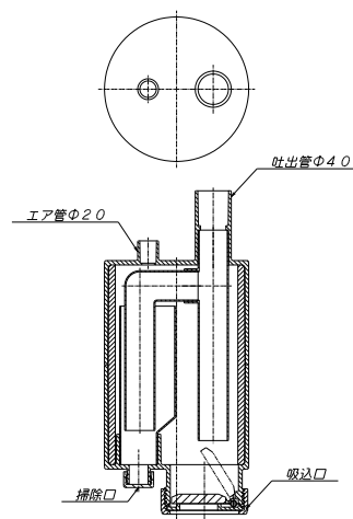
図3 間欠定量移送装置内部構造
