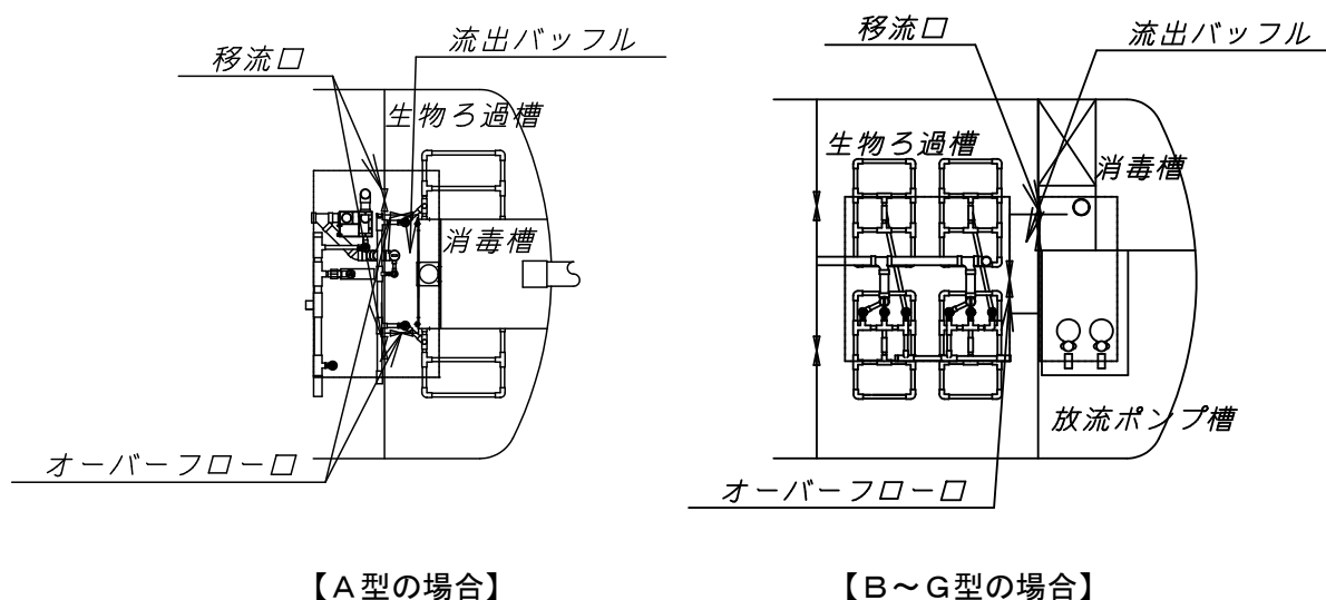
図5. 生物ろ過槽流出バッフル位置
