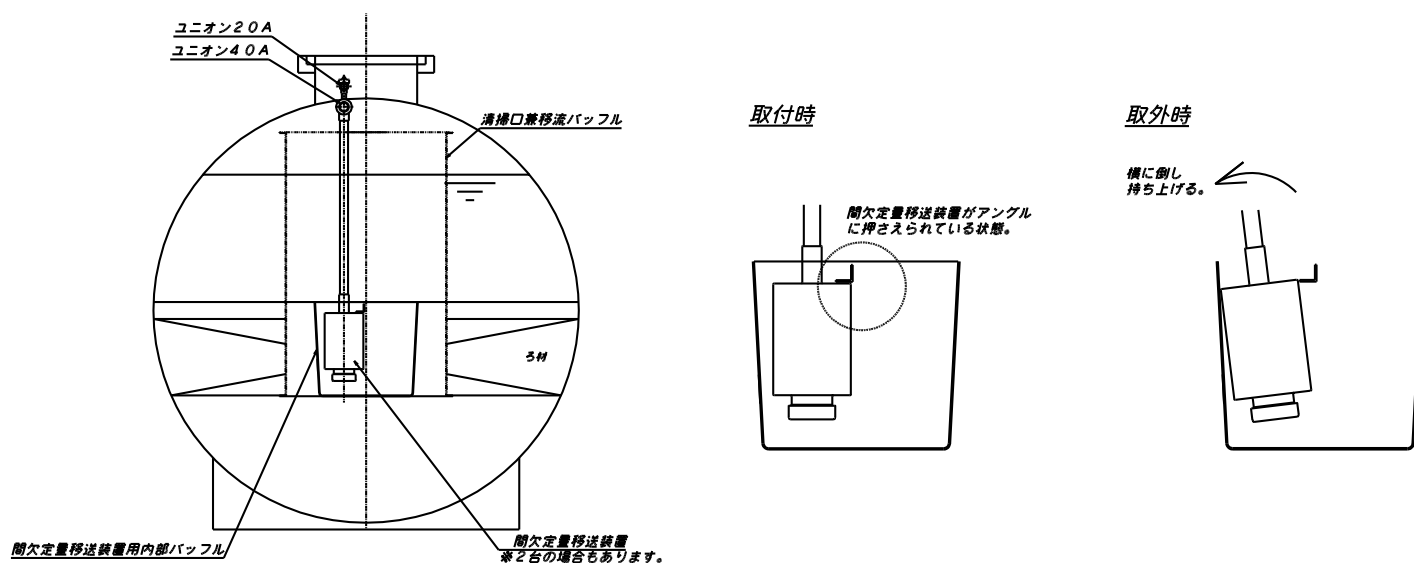
予備ろ過槽移流バッフル部 (DCW-A 型) 断面図
